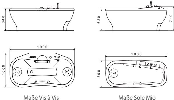
Maße Vis à Vis
