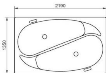
Maße Yin Yang
