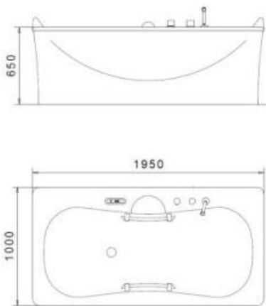
Maße Vis à Vis 1000
