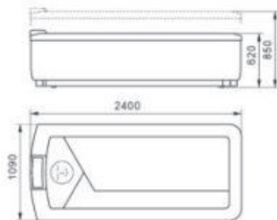
Maße Thermo-Spa Standardverkleidung
