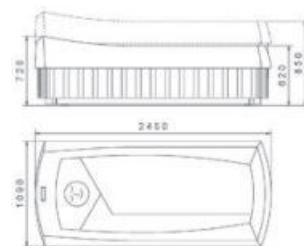
Maße Thermo-Spa Designerverkleidung
