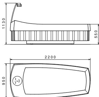
AquaThermoJet dimensions
