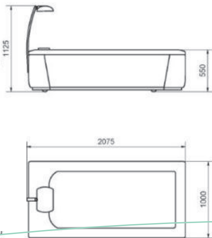
AquaThermoJet dimensions
