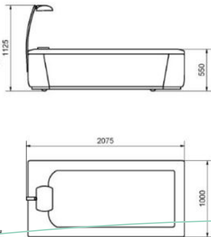
AquaThermoJet dimensions
